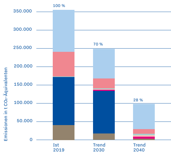
Trend-Szenario (2030, 2040)
