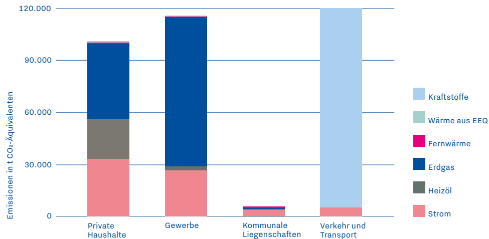
Treibhausgasbilanz 2022
