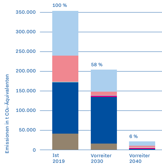
Vorreiter-Szenario 2040
