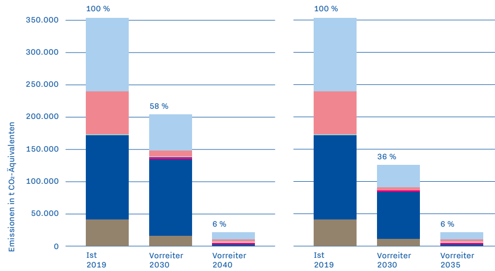
Vorreiter-Szenario 2040
