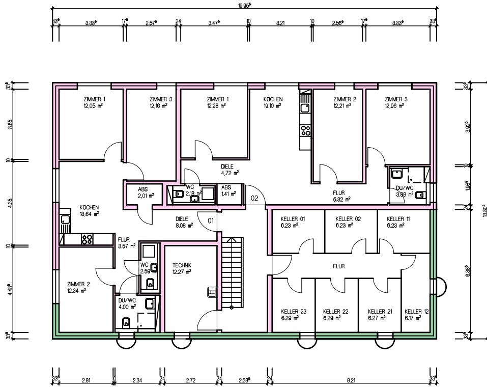
UNTERGESCHOSS
