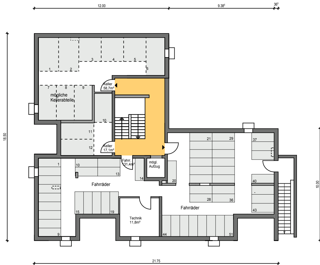
Grundriss Anschlussunterbringung Kellergeschoss
